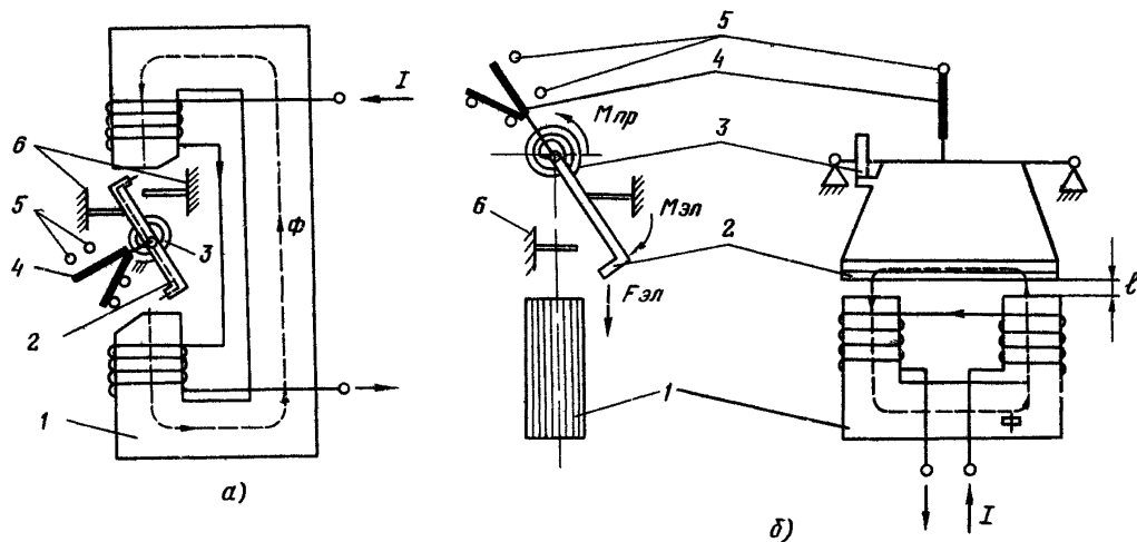
Рис.22. Общий вид электромагнитных систем реле а - серий ЭТ-520 и ЭН-500; б - серий РТ-40 и РН-50; 1 - магнитопровод, 2 - поворотный якорь, 3 - спиральная противодействующая пружина, 4 - подвижной контактный мостик, 5 - неподвижные контакты, 6 - упор
