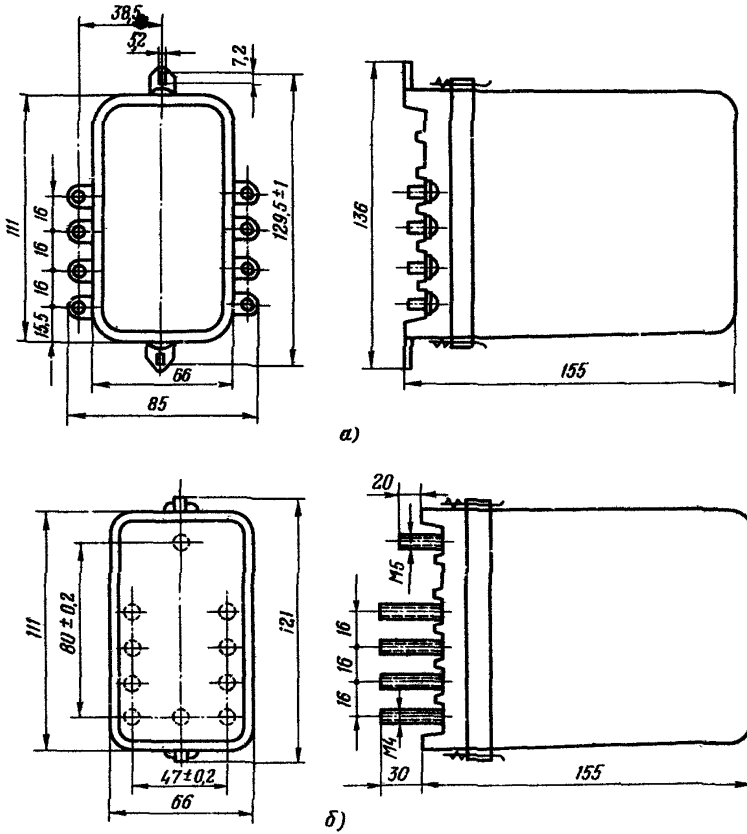
Рис. 5. Габаритные и установочные размеры реле РТ-40, РН-51М, РН-53, РН-54, РН-53/60Д:
