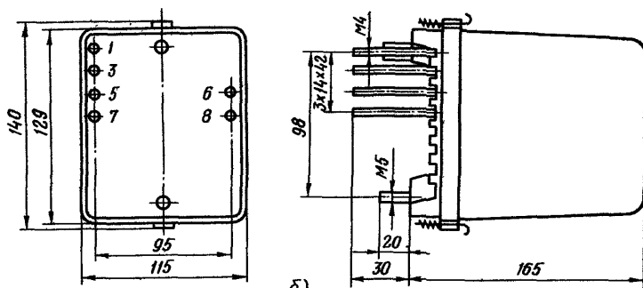
Рис.7. Габаритные и установочные размеры реле РНН-57, РН-58: а - переднее присоединение; б - заднее присоединение.
