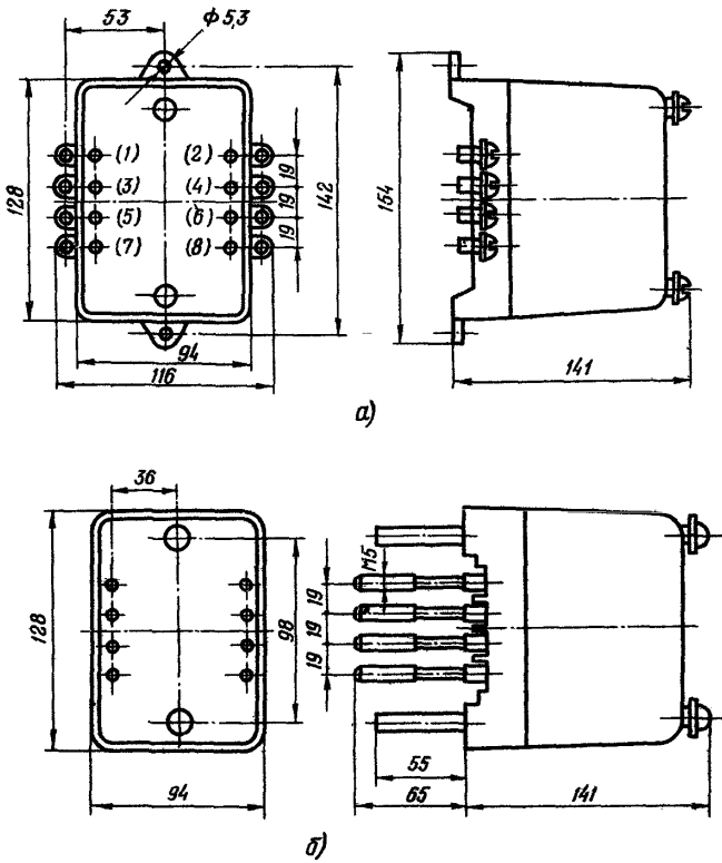
Рис.3. Габаритные и установочные размеры реле ЗТ-520: а - переднее присоединение; б - заднее присоединение
