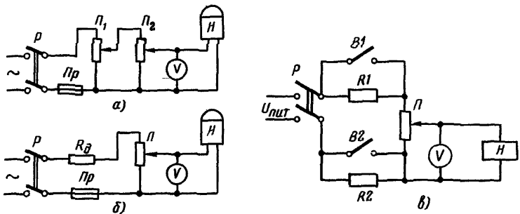
Рис. 17. Схемы для настройки реле ЭН и РН с малыми пределами уставок: а - с двумя потенциометрами \Pi_1 и \Pi_2 ; б - с потенциометром \Pi и добавочным резистором R_2 ; в - с автотрансформатором AT и потенциометром \Pi
