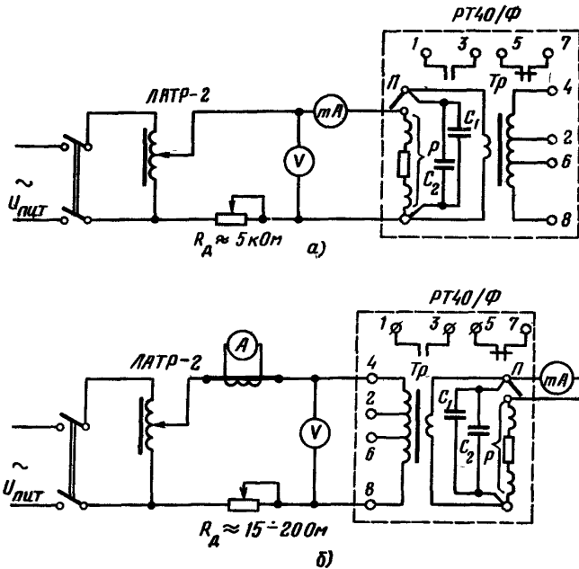
Рис. 18. Схемы для проверки и настройки реле РТ-40/Ф: а - схема для проверки токов и напряжения срабатывания и возврата при подаче тока в обмотку; б - схема для проверки реле РТ-40/Ф при подаче питания в первичную обмотку трансформатора реле
