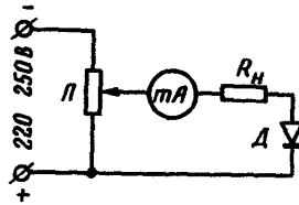
Рис. 19. Схема для дополнительной проверки диодов типа Д-226
