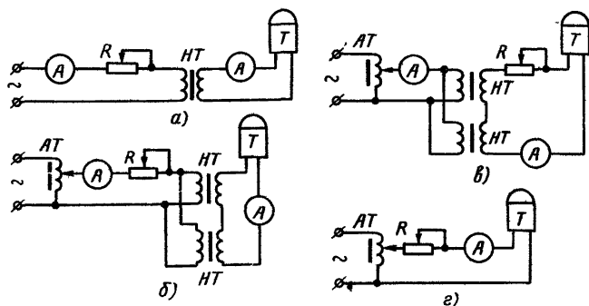
Рис. 15. Схемы регулирования тока реле с нагруженными трансформаторами и автотрансформаторами:
