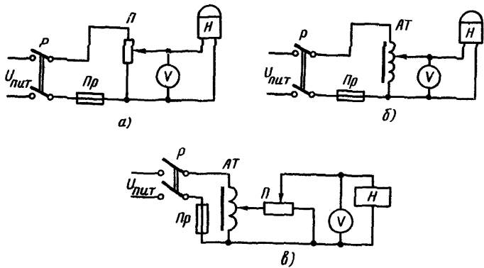
Рис. 16. Схемы регулирования напряжения: а - с потенциометром \Pi ; б - с автотрансформатором AT ; в - с двумя резисторами и потенциометром
