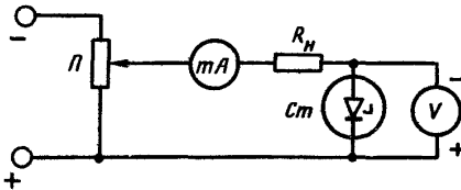
Рис.21. Схема для проверки стабилитрона Д-806
