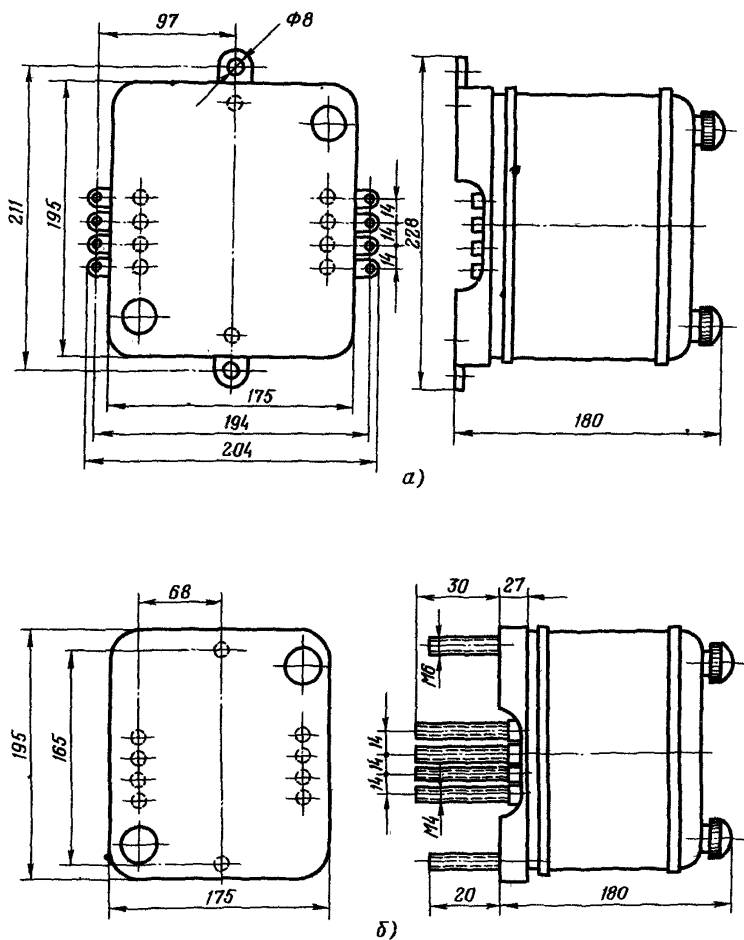
Рис.6. Габаритные и установочные размеры реле РТ-40/Ц, РТ-40/Ф, РТ-40/Р:
