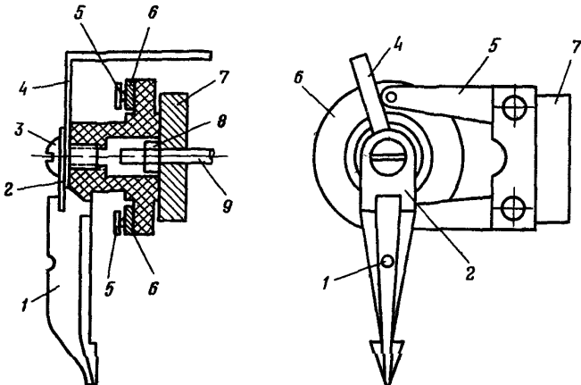
Рис. 12. Регулировочная головка реле Э-520 (нового выпуска):
