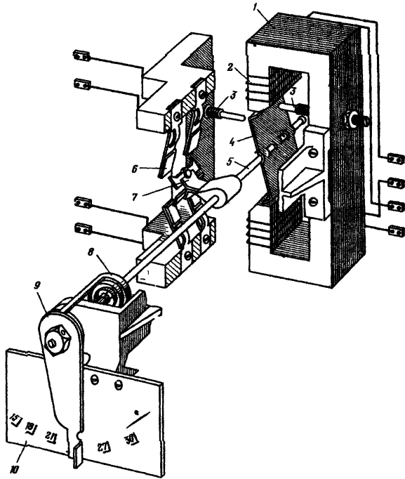
Рис.23. Кинематическая схема реле 3-520:
