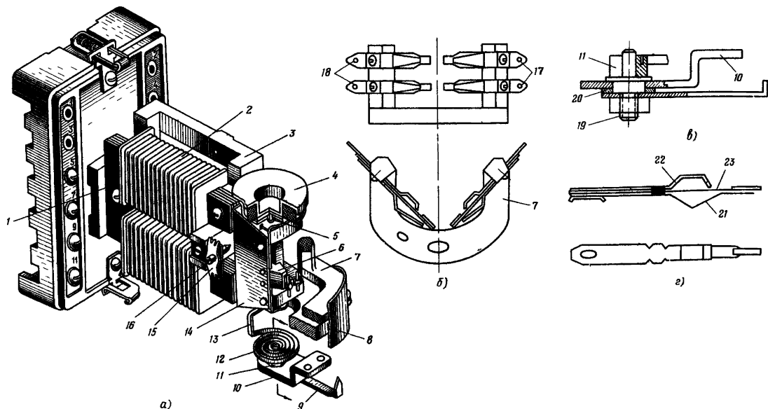
Рис. 13. Общий вид реле РТ-40 (РН-50):
