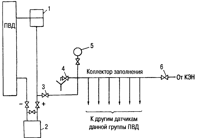
Схема организации заполнения импульсных линий датчиков уровнемеров ПВД посторонним конденсатом:
