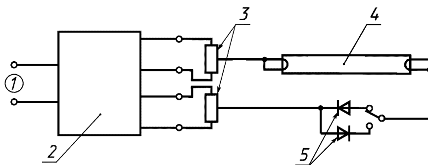
1 — сеть; 2 — испытываемый ПРА; 3 — резистор; 4 — лампа; 5 — выпрямитель
