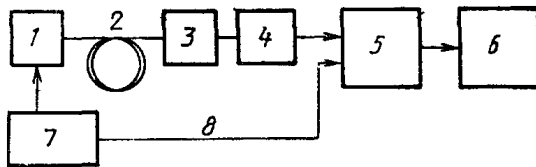
1 — лазерные диоды; 2 — испытуемое волокно; 3 — аттенюатор; 4 — оптический детектор; 5 — векторный вольтметр; 6 — ЭВМ; 7 — генератор импульсов; 8 — контрольный сигнал
