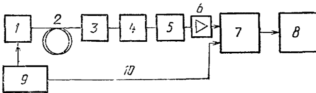
1 — светодиоды; 2 — испытуемое волокно; 3 — селектор длины волны; 4 — аттенюатор; 5 — оптический детектор; 6 — усилитель; 7 — векторный вольтметр; 8 — ЭВМ; 9 — генератор импульсов; 10 — контрольный сигнал
