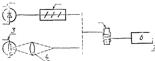
Аппаратура для измерения затухания на установленной длине волны
