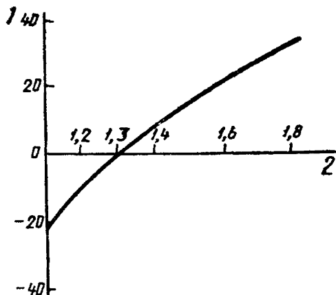
Коэффициент хроматической дисперсии в зависимости от длины волны
