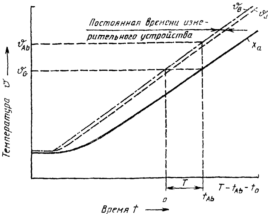
Рисунок ВВ1 — Определение постоянной времени методом быстрого изменения температуры
