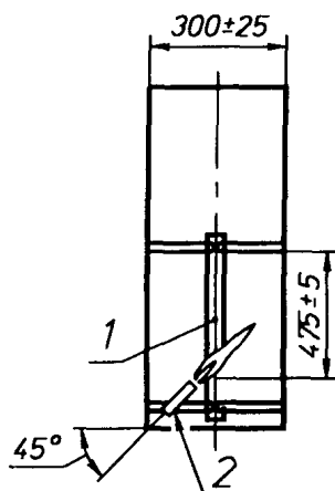
Рисунок 3 — Расположение горелки мощностью 1 кВт относительно образца
