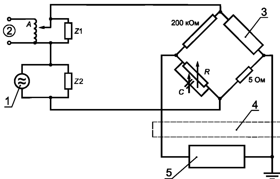
Рисунок А.1 — Измерение токов
