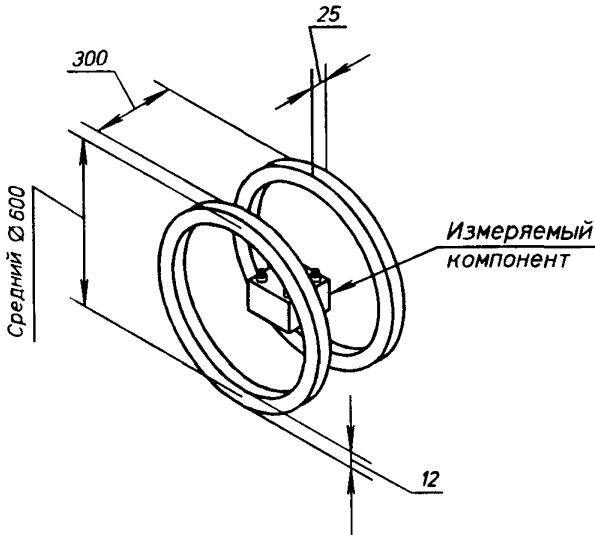
Рисунок 22 — Кольца Гельмгольца
