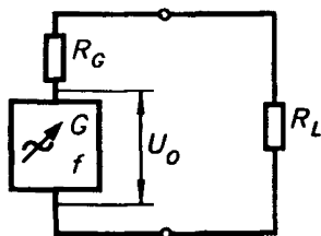
Рисунок 17 — Иллюстрация потерь от несогласования
