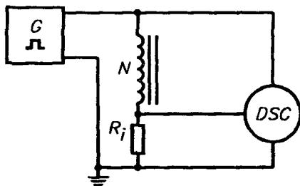
Рисунок 19 — Схема для проверки произведения напряжения на время (измерение осуществляется без подмагничивания и с использованием одиночных импульсов)
