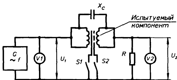
Рисунок 10 — Схема для определения межобмоточной емкости
