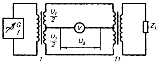
TI — испытуемый трансформатор
