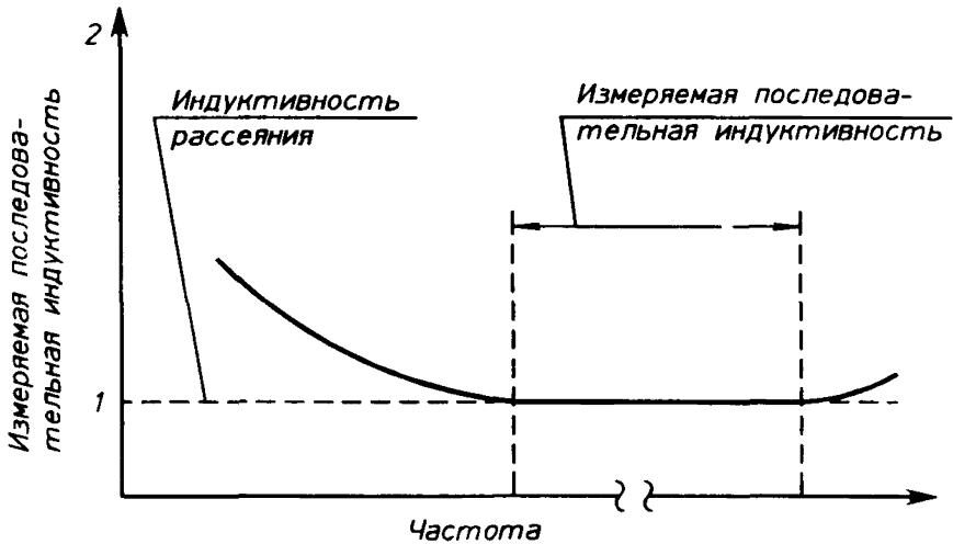
Рисунок 4 — Зависимость измеряемой последовательной индуктивности от частоты
