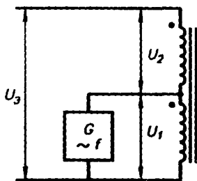
Рисунок 21 — Проверка фаз (полярности) путем измерения напряжений
