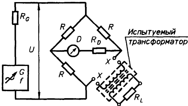
Рисунок 18 — Основная испытательная схема для измерения потерь от несогласования
