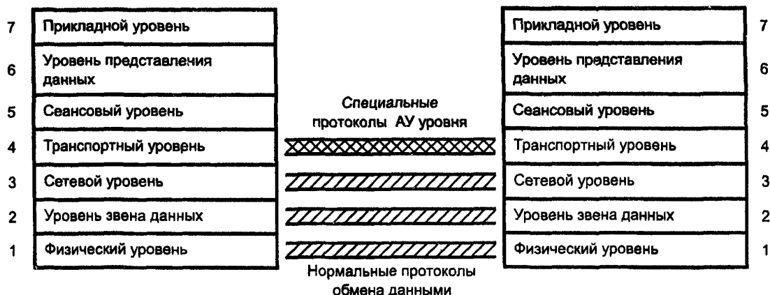
Рисунок А.2 — Обмен АУ (N)-уровня
