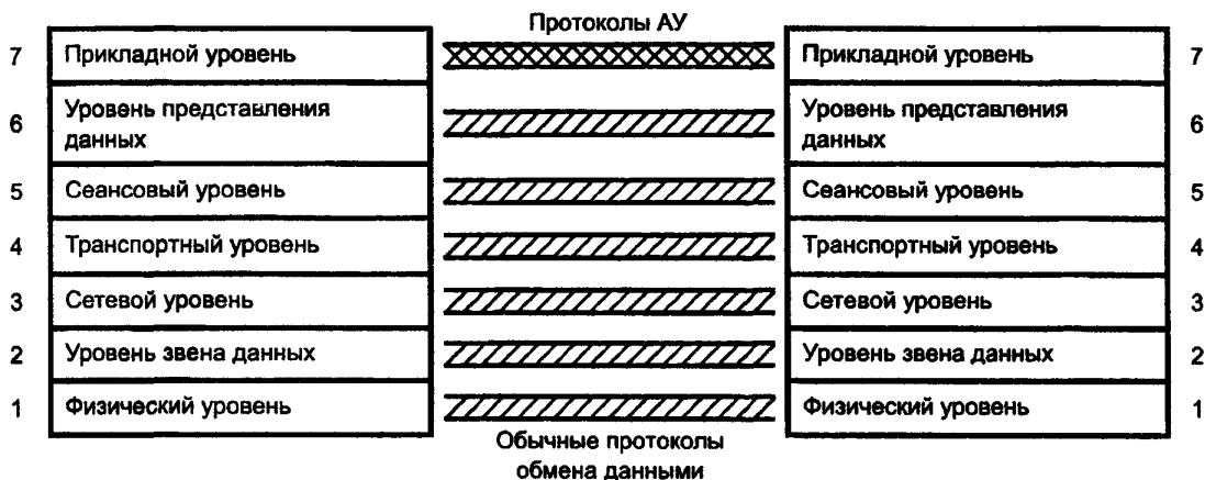
Рисунок А.1 — Обмен информацией АУ систем
