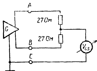
Рисунок 8 Измерение смещения напряжения
