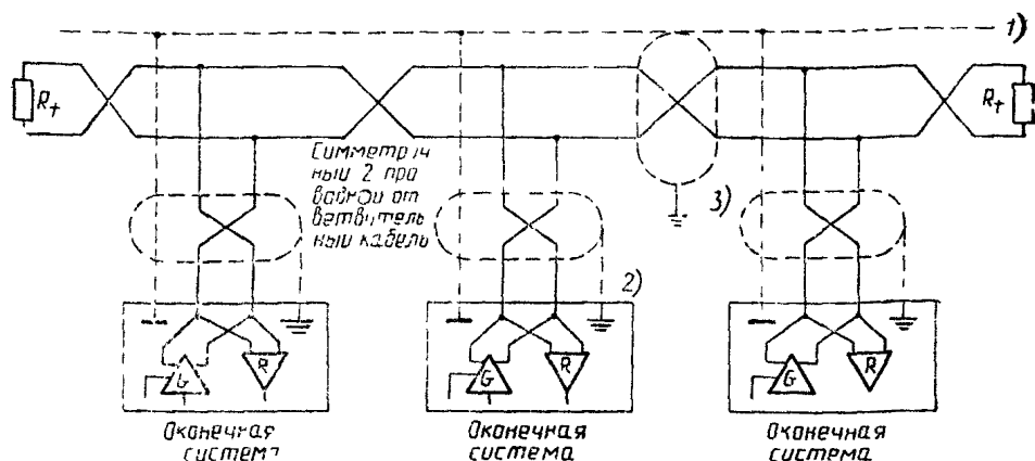
Рисунок 2 Двухпроводная многопунктовая конфигурация
