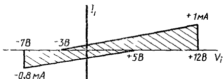
Рисунок 4 Ограничения тока 1,0 ЕН
