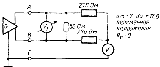
Рисунок 9 Измерение напряжения нагруженного выхода
