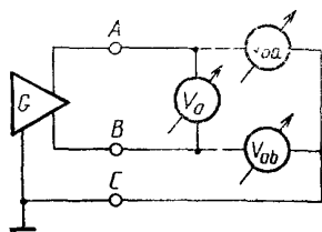
Рисунок 7 Измерение напряжения разомкнутой цепи
