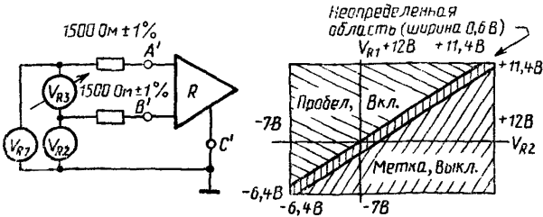
Рисунок 12 Измерение рассогласования на входе
