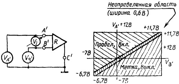
Рисунок 11 Диапазон входных напряжений
