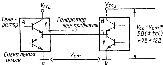
Рисунок 16 Соперничество генераторов с одним генератором-источником
