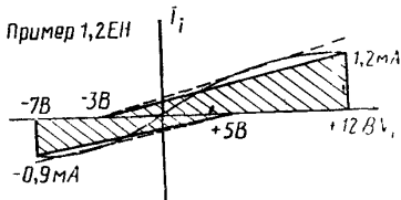
Рисунок 6 Определение значения ЕН
