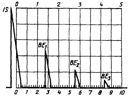
Удовлетворительное соединение
