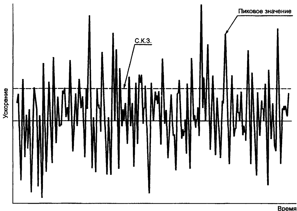
Рисунок А.2 — Отсечка (ограничение) сигнала
