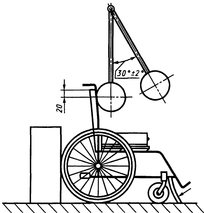
Рисунок 16 — Испытание спинки кресла-коляски на ударную прочность
