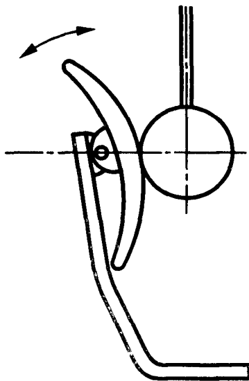
Рисунок 15 — Спинка кресла-коляски с самонастраивающимся углом наклона
