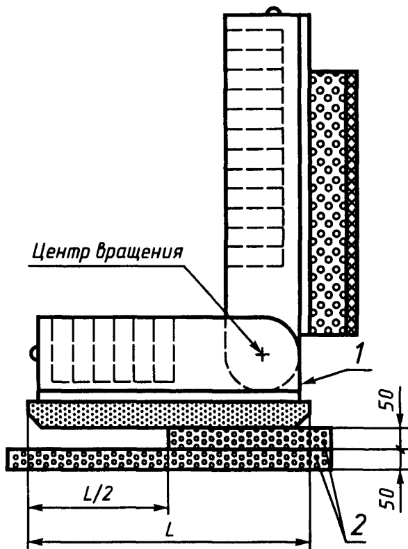
1 — испытательный манекен; 2 — пенопластовые прокладки
