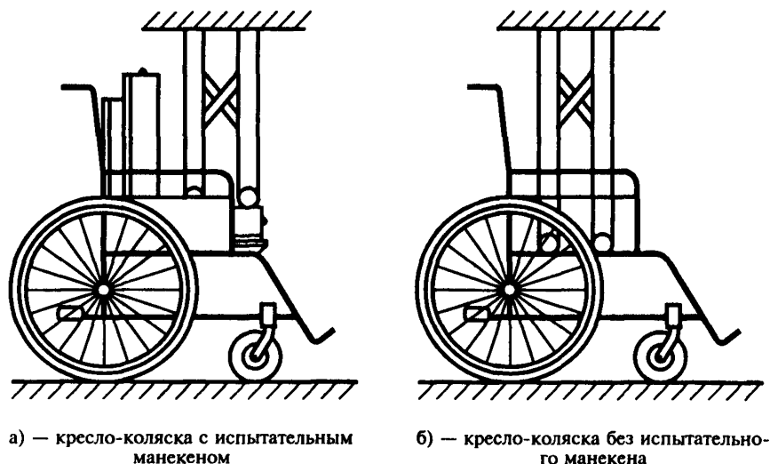
Рисунок 6 — Устройство, удерживающее кресло-коляску от опрокидывания
