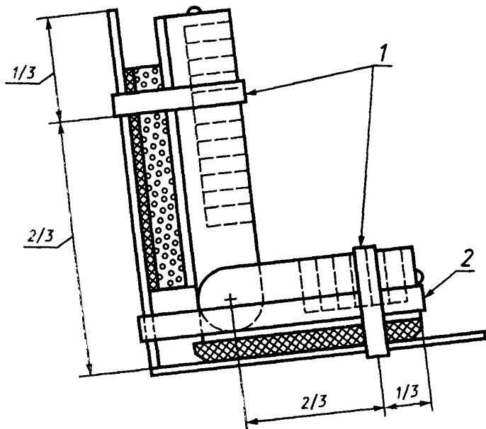
Рисунок 17 — Расположение ограничителей для проведения испытаний на усталостную прочность
