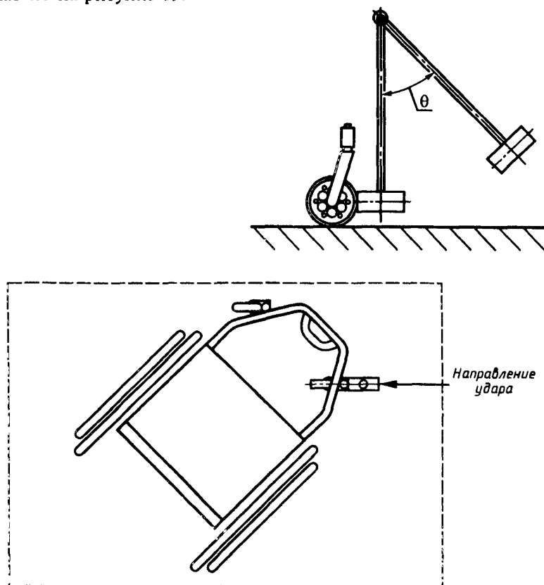
Рисунок 19 — Испытания поворотных колес кресла-коляски на ударную прочность
