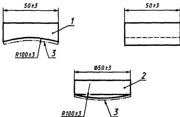
Рисунок 1 — Нагружающие пластины
