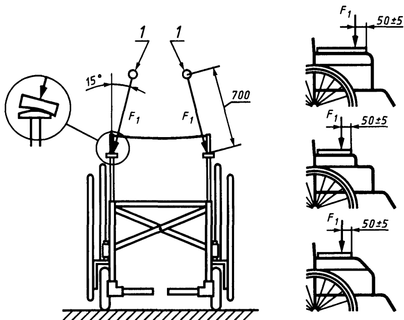
1 — точка приложения испытательной нагрузки
