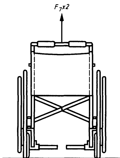
б) — кресло-коляска с ручкой, состоящей из одной поперечной перекладины
