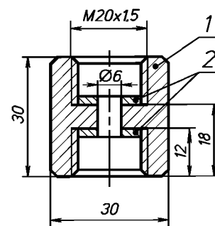
1 — переходник; 2 — прокладка
