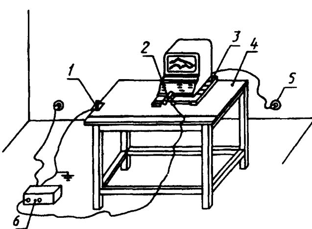
1 – зажим; 2 – разрядное устройство; 3 – изолирующая плоскость; 4 – эталонная плоскость земли; 5 – сетевая розетка; 6 – генератор ЭСР
