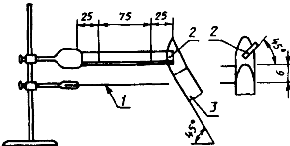
1 – металлическая (проволочная) сетка; 2 – образец; 3 – горелка
