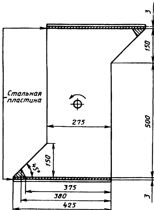
Рисунок 21.101 — Вращающийся барабан
