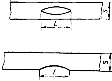
Рисунок 2 — Длина дефекта
