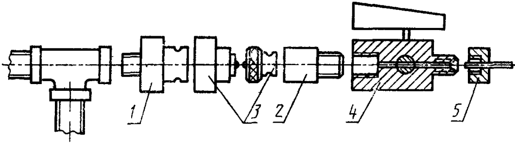
1 — запорный клапан, постоянно подсоединенная часть быстроразъемного соединения; 2 — съемная часть быстроразъемного соединения (если применяется); 3 — защи. ные крышки, 4 — сферический край, 5 — насадок
