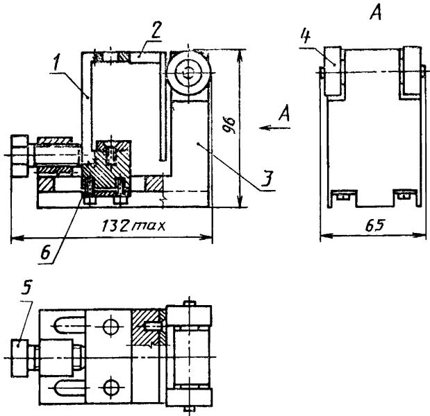
1 — ползун; 2 — прижим; 3 — корпус; 4 — ролик; 5 — регулировочный винт; 6 — шайба
