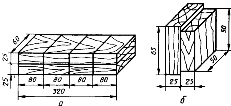
а — склеенные бруски; б — образец для испытания
