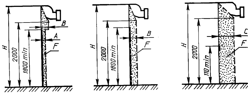
а) жесткое ограждение б) сетка или экран в) ограждение с поручнями, цепями или канатом
