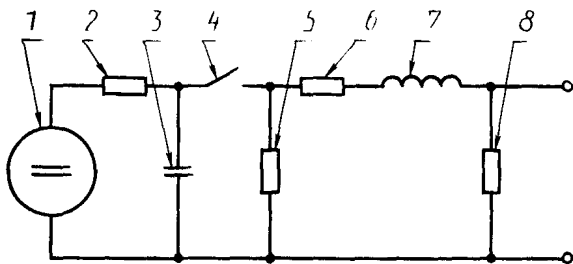
Упрощенная схема ИГ МИП
