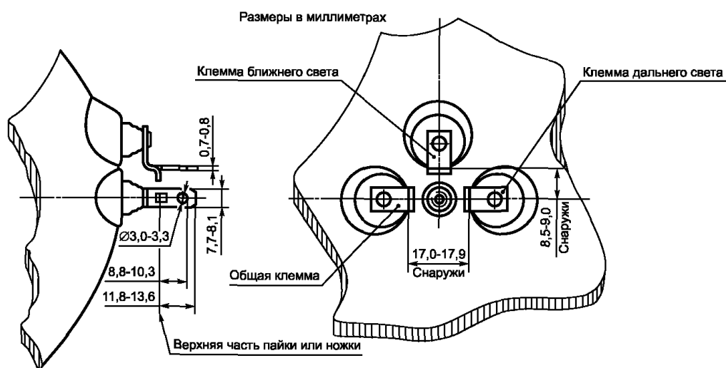
Категория 22 (ближнего и дальнего света)
