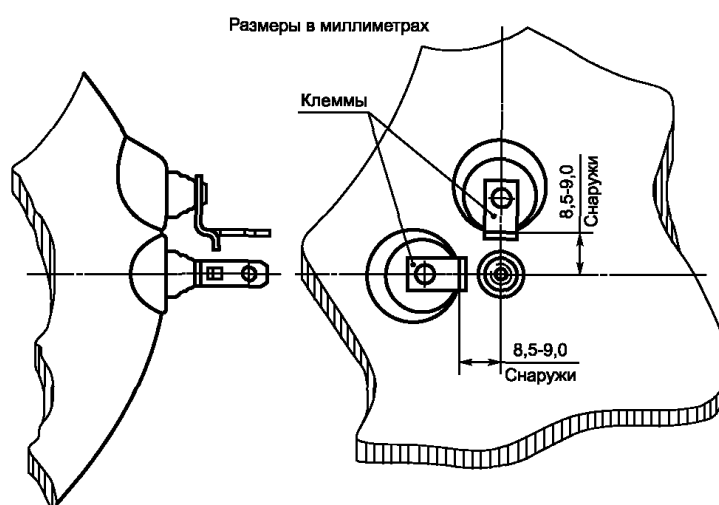
Категория 21 (только ближнего света)
