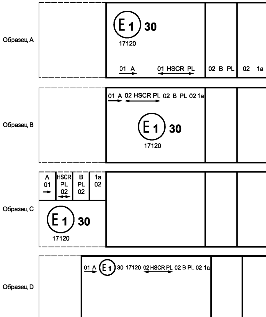
Рисунок 8 — Упрощенная маркировка сгруппированных, комбинированных или совмещенных огней
