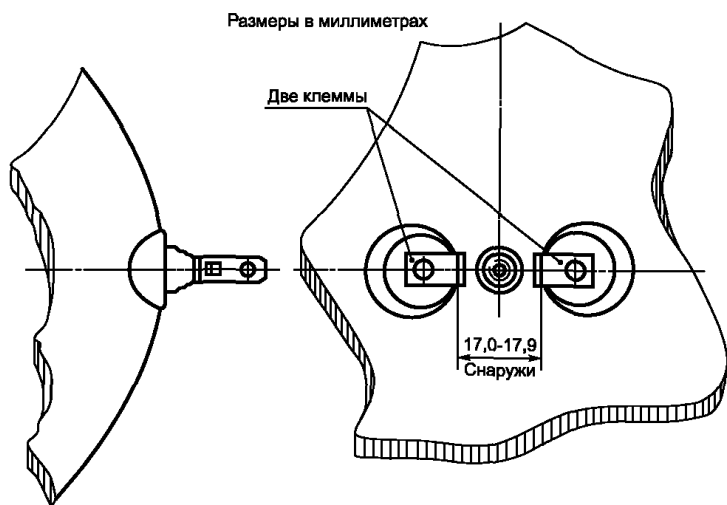
Категория 1 (только дальнего света)
