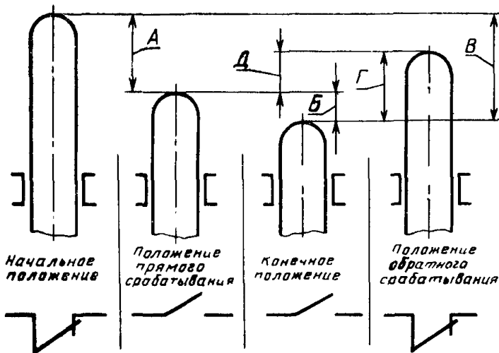
Схема положения подвижных частей выключателя
