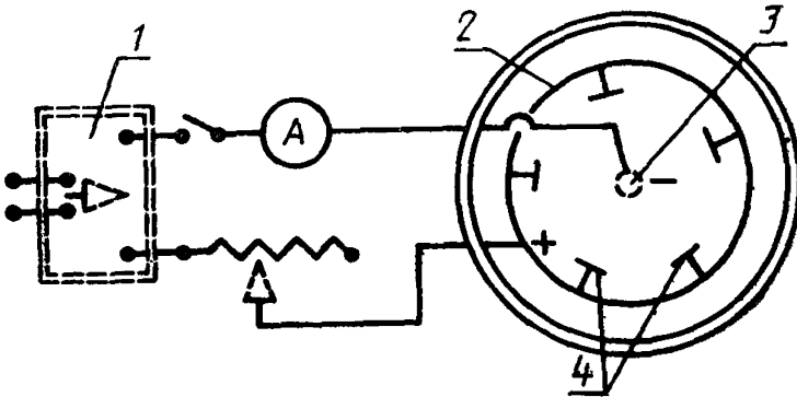
Схема установки катодной очистки пластин
