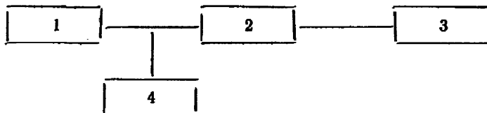
1—источник постоянных напряжений; 2—образцовый делитель напряжения; 3—поверяемый вольтметр; 4—образцовый вольтметр (потенциометр)
