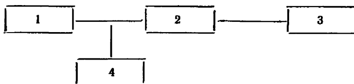
1—источник постоянных напряжений; 2—образцовый делитель напряжения; 3—образцовый вольтметр (потенциометр); 4—поверяемый вольтметр
