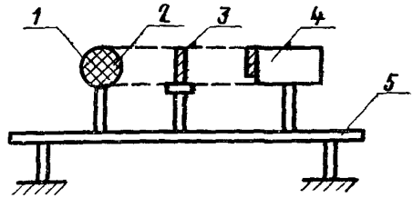
1 — изотопный источник быстрых нейтронов, 2 — шаровой замедлитель, 3 — кадмиевый экран, 4 — блок детектирования, 5 — градуировочная линейка
