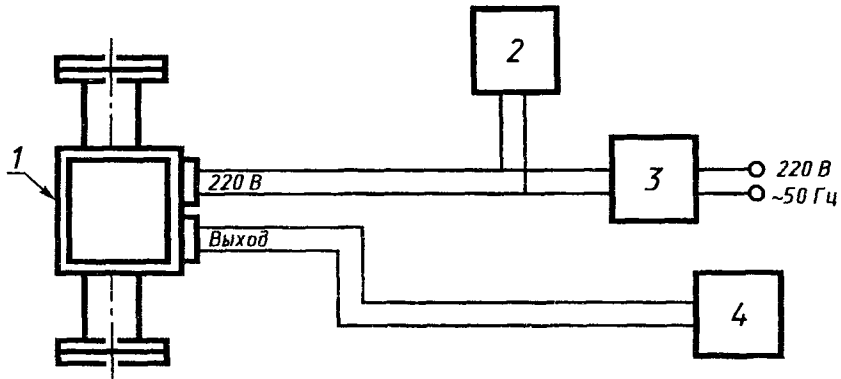
Схема подключения питания к ротаметру
