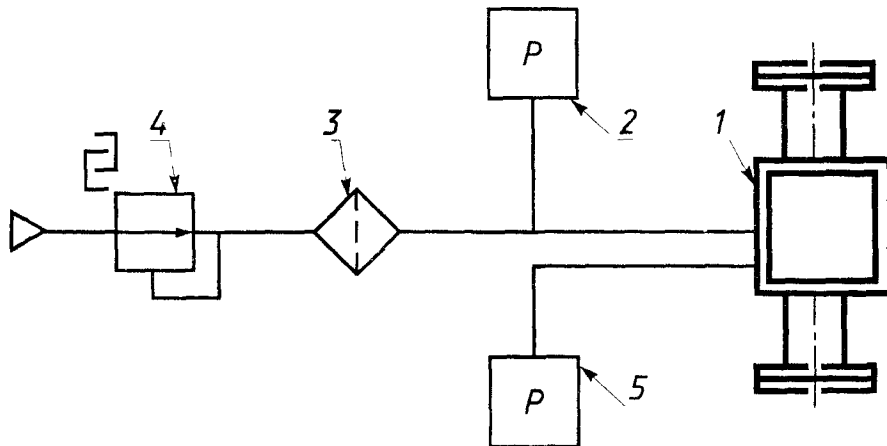
Схема подключения к ротаметру линии пневматической связи
