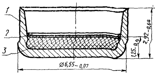
1 — колпачок, 2 — кружок, 3 — состав ударный Черт. 1
