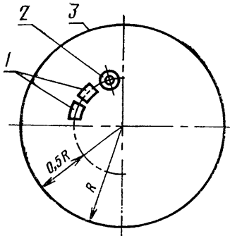
Схема вырезки образцов для механических испытаний
