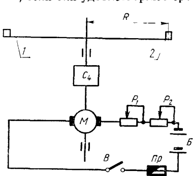
1—крестовина, 2—стойка для крепления анемометров, C_4 —счетчик частоты вращения крестовины, M —двигатель; P_1 , P_2 —реостаты, B —аккумуляторная батарея; B —выключатель, Pr —предохранитель
