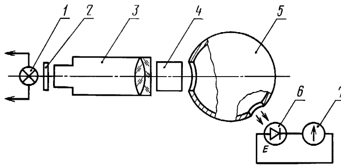
1 — источник света; 2 — диафрагма; 3 — коллиматор, дающий параллельный пучок лучей; 4 — испытуемый объектив; 5 — фотометрический шар; 6 — фотоэлектрический приемник; 7 — гальванометр
