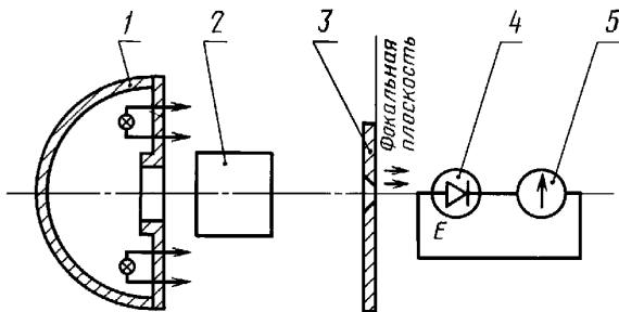
1 — осветитель; 2 — испытуемый объектив; 3 — диафрагма; 4 — фотоэлектрический приемник; 5 — гальванометр
