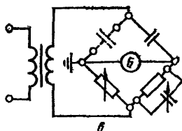
Схема с заземленной диагональю
