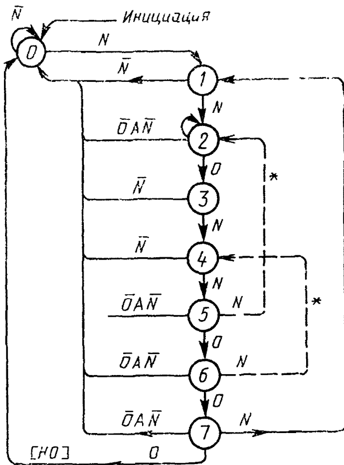
Конечный автомат обнаружения молч/раб
