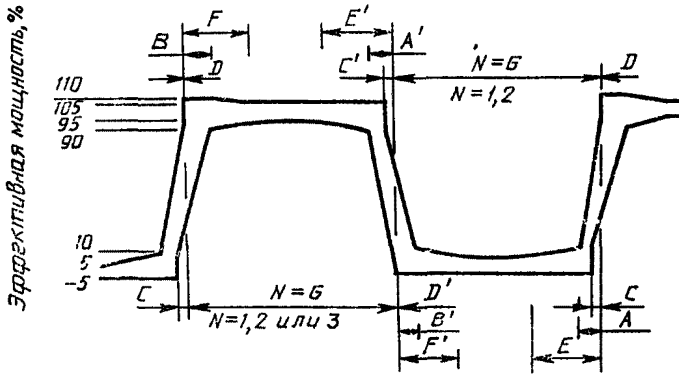
Форма оптического волнового сигнала
