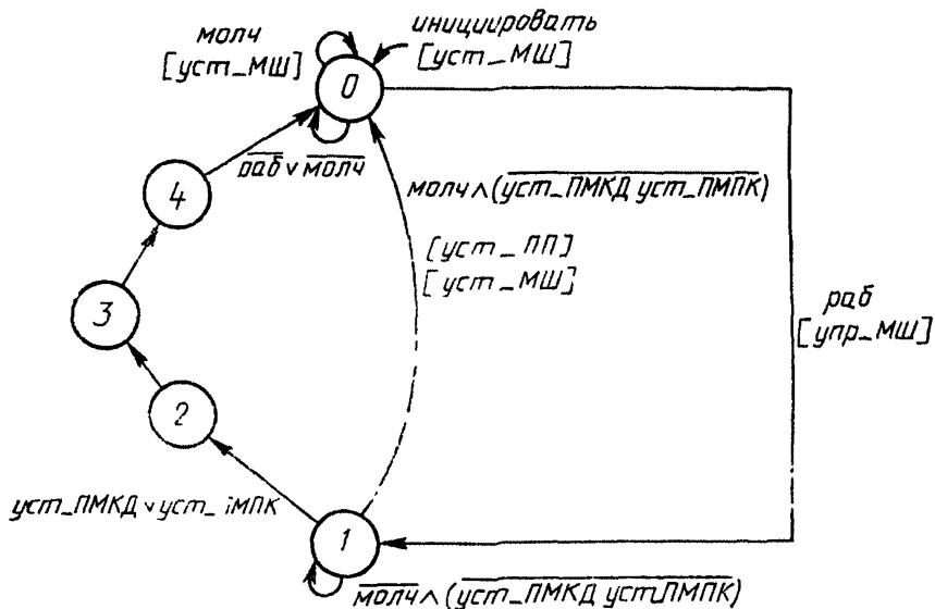
Конечный автомат пакет_помех/молчание_шины
