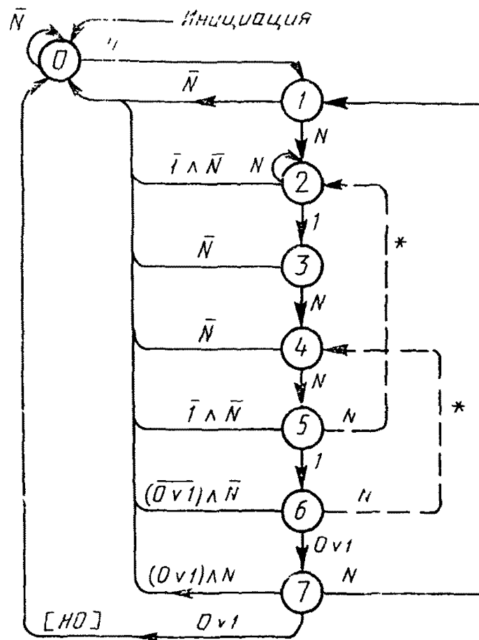
Конечный автомат обнаружения ОК
