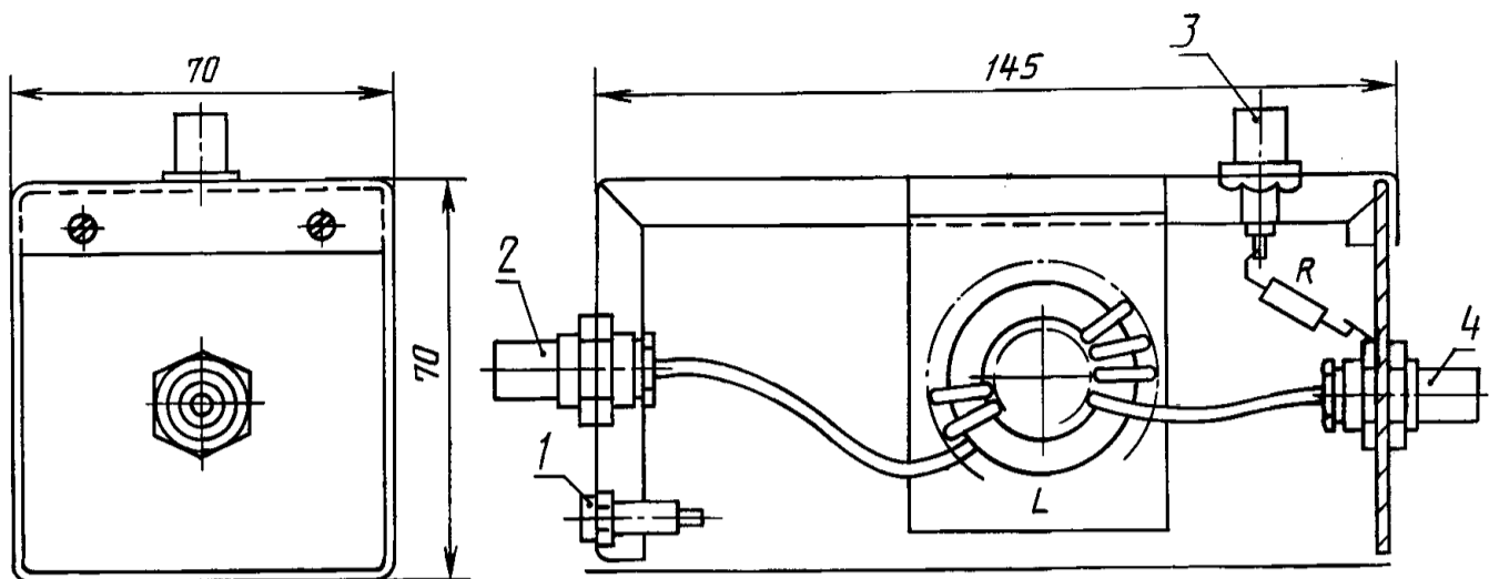
1 — зажим заземления; 2 — разъем подключения полезного сигнала (цепь генератора телевизионных испытательных сигналов); 3 — разъем подключения источника помех (цепь ВЧ генератора); 4 — разъем подключения испытуемого ВМ; R = 100 \text{ Ом} ; L = 30 \text{ мкГн}
