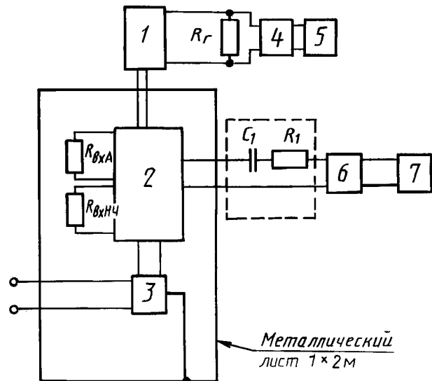
Схема проведения испытаний на устойчивость ВМ к наведенным ВЧ напряжениям на выходных звуковых зажимах
