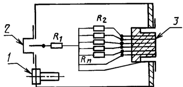
1 — зажим заземления; 2 — разъем подключения источника помех (цепь ВЧ генератора); 3 — разъем подключения испытуемого ВМ; R_1 = 100 \text{ Ом} ; R_2 \dots R_n составляют: 2 \times 2,2 \text{ кОм} — для магнитного звукоснимателя; 2 \times 470 \text{ кОм} — для кристаллического звукоснимателя; 2 \times 47 \text{ кОм} — для тюнера; 4 \times 47 \text{ кОм} — для звуковой вх/вых
