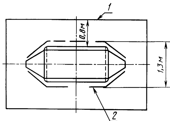
Схема расположения открытой Т-камеры в экранированном помещении
