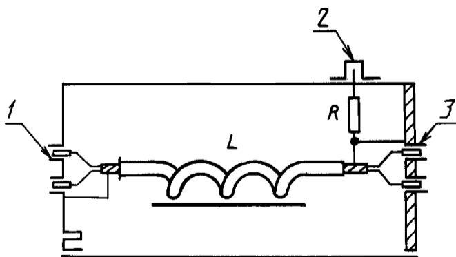
1 — разъем подключения входных или выходных звуковых сигналов; 2 — разъем подключения источника помех (цепь ВЧ генератора); 3 — разъем подключения испытуемого ВМ; L = 30 \text{ мкГн} ; R = 100 \text{ Ом}
