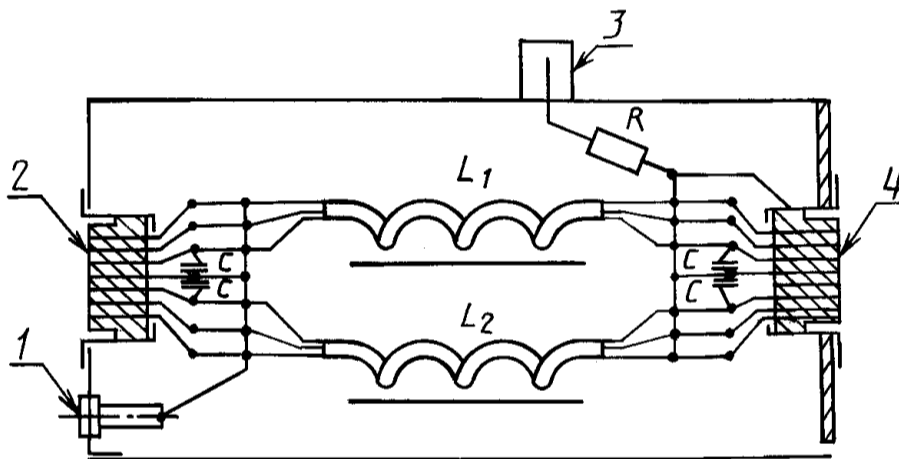
1 — зажим заземления; 2 — разъем подключения полезного сигнала (цепь генератора телевизионных испытательных сигналов); 3 — разъем подключения источника помех (цепь ВЧ генератора); 4 — разъем подключения испытуемого ВМ; C = 1 \text{ нФ} ; L_1 = L_2 = 60 \text{ мкГн} ; R = 100 \text{ Ом}
