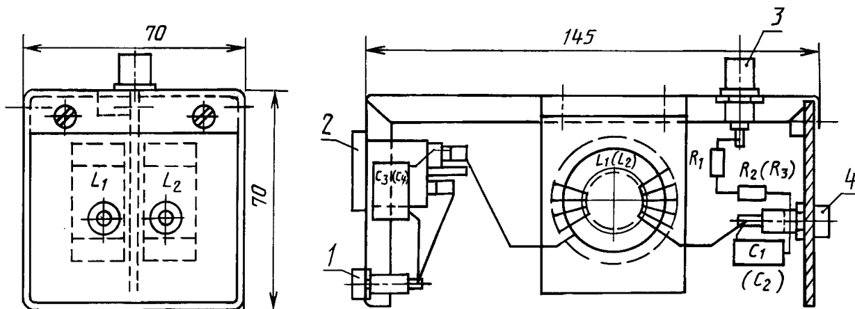
Блок связи типа М. Сборочный чертеж
