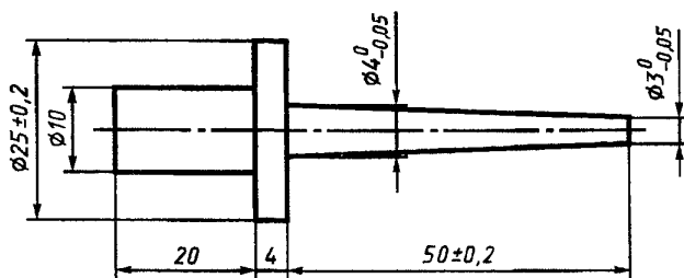
Рисунок 101 — Длинный испытательный стержень
