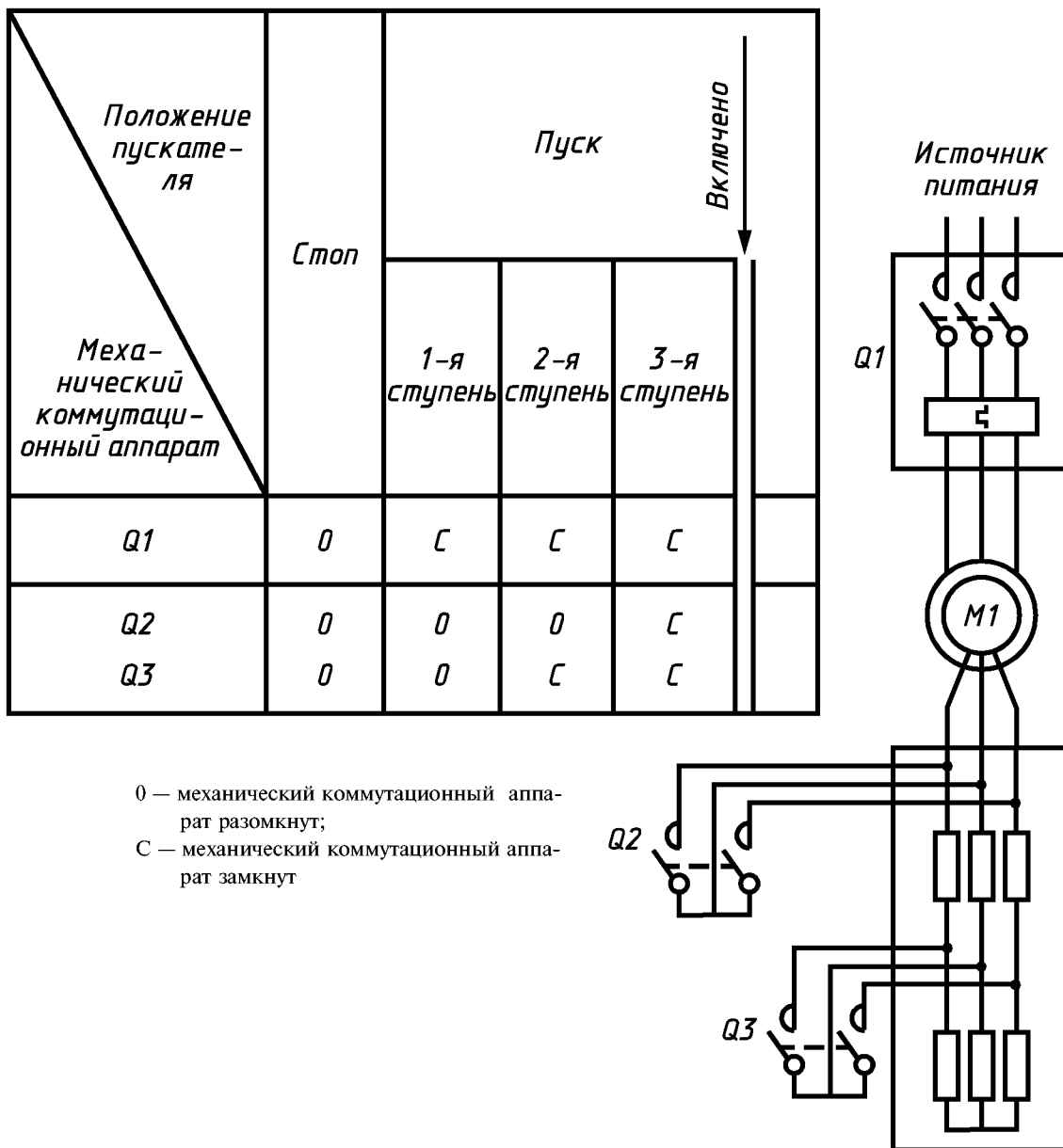
Рисунок 4 — Пример схемы трехфазного реостатного роторного пускателя с тремя пусковыми ступенями (2.2.16) и одним направлением вращения (в случае, если все механические коммутационные аппараты представляют собой контакторы)
