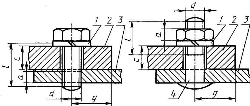
1 — блокирующее устройство; 2 — кабельный наконечник или шина; 3 — фиксируемая часть; 4 — болт
