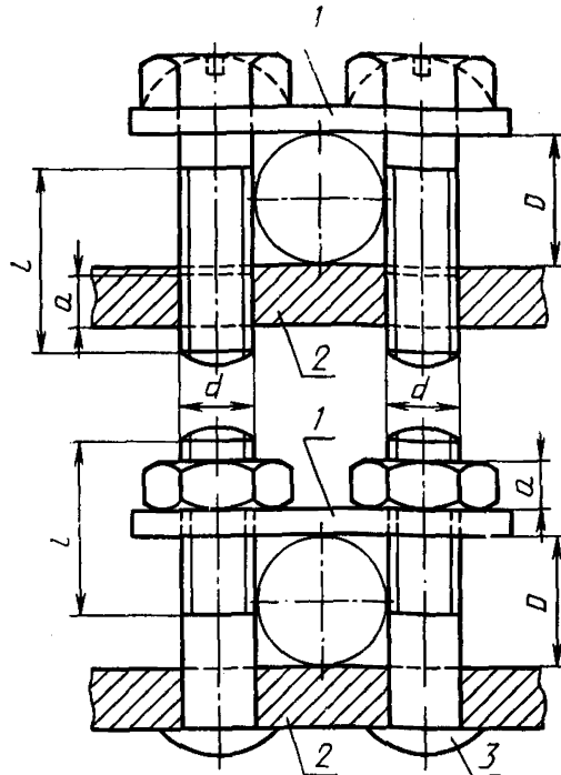
1 — прижимная планка; 2 — фиксируемая часть; 3 — болт
