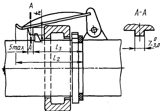
Размеры, мм
