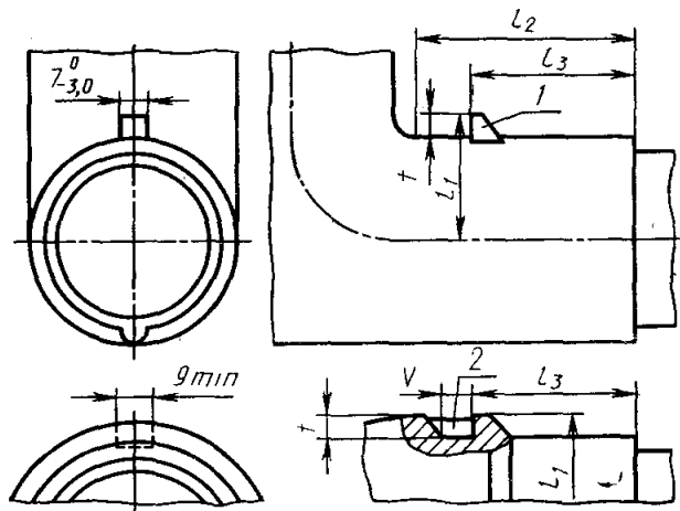
1 — выступ; 2 — выемка
