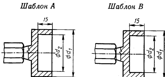
Калибр для проверки диаметра d_2
