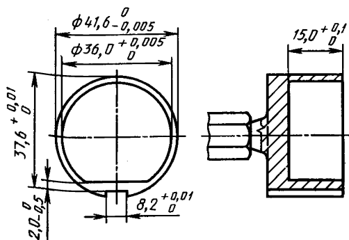
Калибр Б
