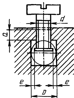
Зажим без прижимной пластины
