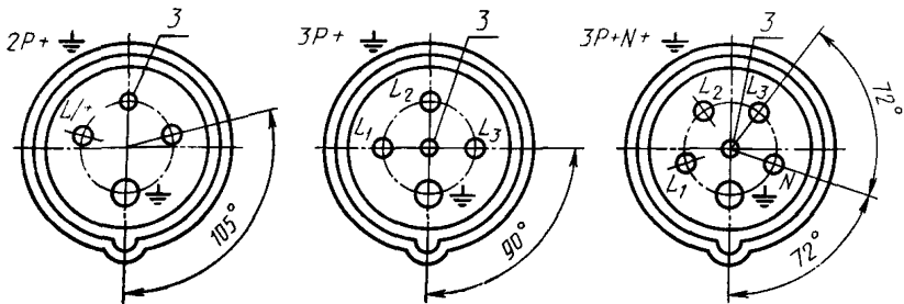
Расположение контактных гнезд
