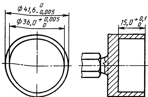
Калибр Б
