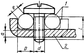
Винт, не требующий шайбы или прижимной пластины
