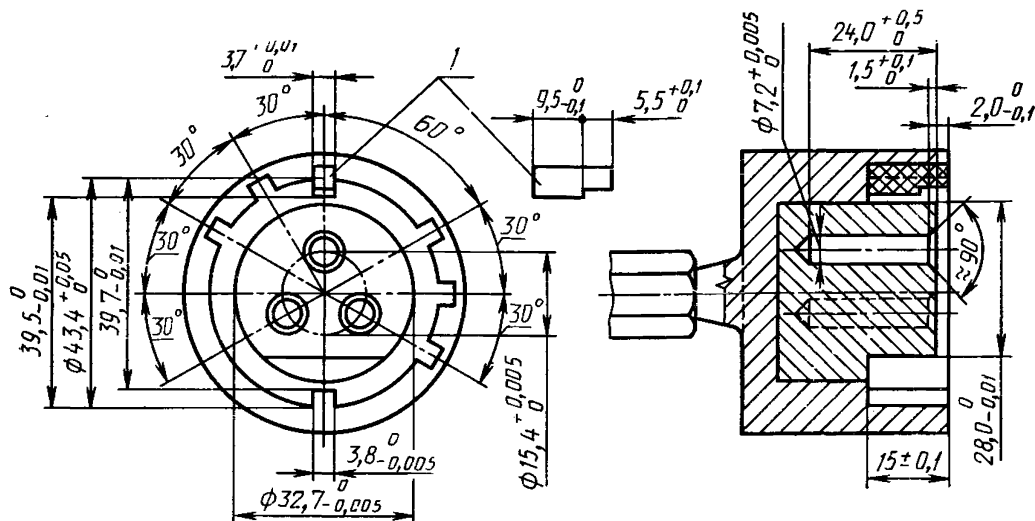
Размеры, мм
