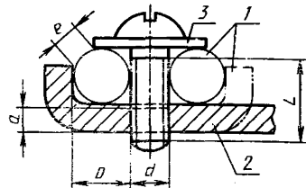
Винт, требующий шайбу или прижимную пластину
