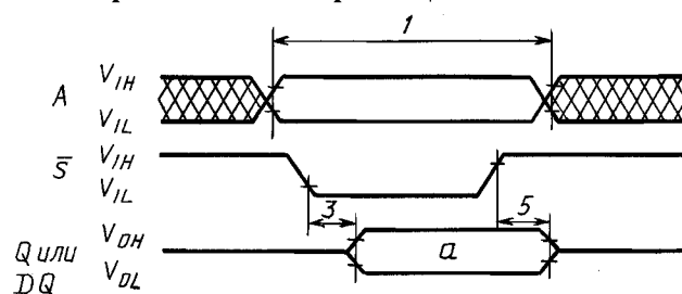
Типовое статическое запоминающее устройство с произвольной выборкой. Цикл считывания
