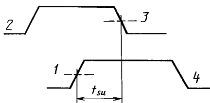
Время установления (типичные формы сигнала)
