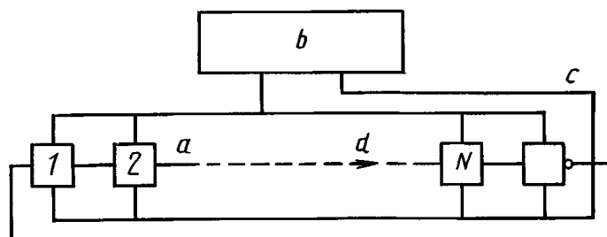
Кольцевой генератор для неинвертирующих N-схем
