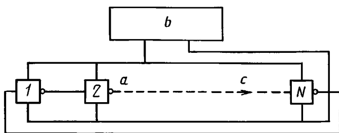
Кольцевой генератор для инвертирующих N-схем
