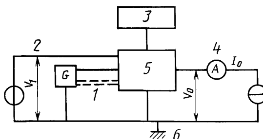
G — источник напряжения и генератор импульсов; 1 — другие входы; 2 — измеряемый вход; 3 — источник питания; 4 — измеряемый выход; 5 — измеряемая схема; 6 — опорная шина
