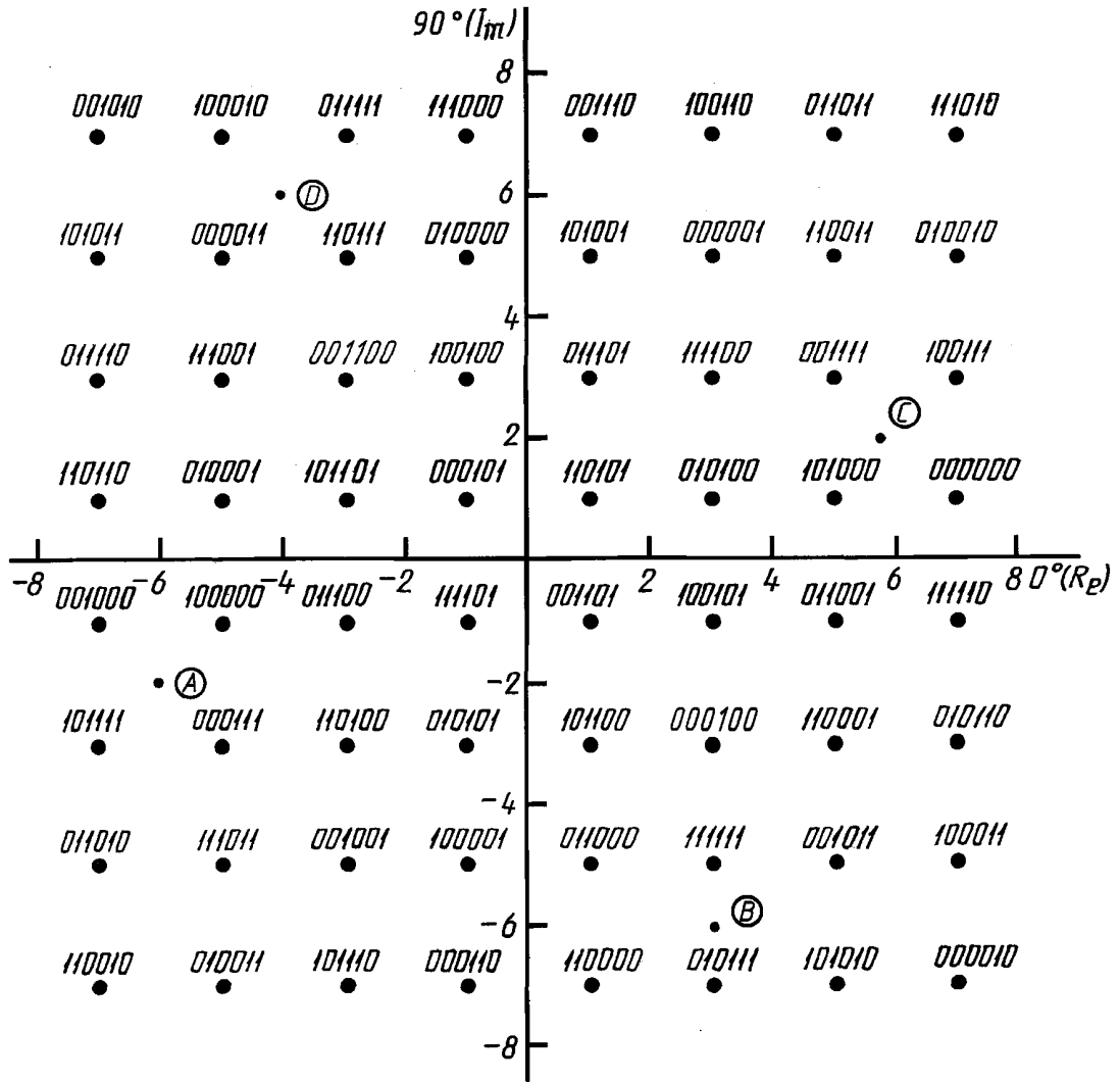
Сигнальное созвездие для скорости 12000 бит/с
