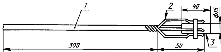
Рисунок 3 — Устройство для взятия навески
