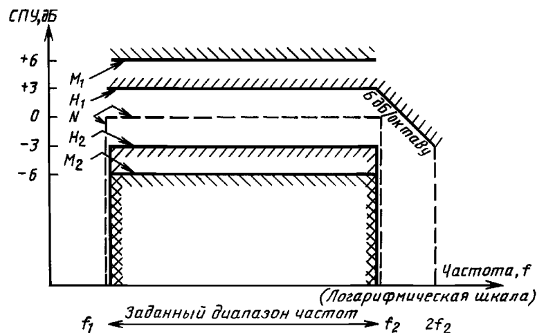
Спектр плотности ускорения (СПУ) и границы допусков
