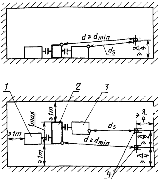
1 — приводной узел; 2 — редуктор; 3 — нагрузочный узел; 4 — микрофон
