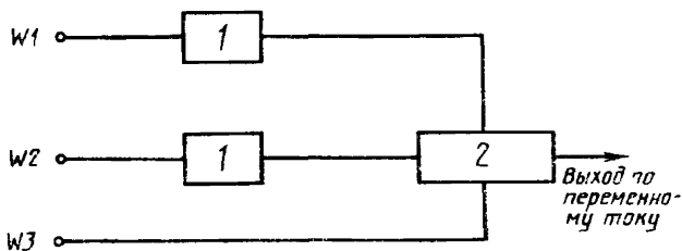
1 — единица СБП; 2 — переключающее устройство
