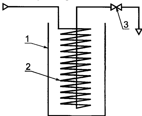
Устройство для охлаждения сжиженного углеводородного газа
