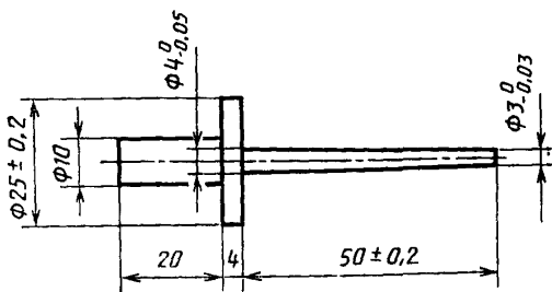
Длинный испытательный палец
