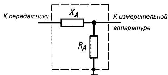
R_A, X_A — параметры эквивалента антенны
