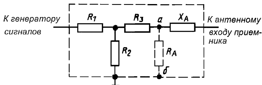
R_A, X_A — параметры эквивалента антенны
