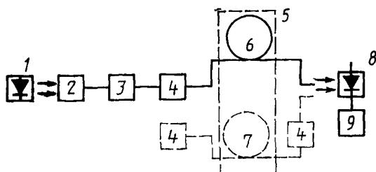
1—источник излучения; 2—устройство ввода; 3—сместитель мод; 4—фильтр мод оболочки; 5—измеряемый кабель; 6—оптическое волокно, подверженное влиянию; 7—влияющее волокно; 8—приемник излучения; 9—регистрирующее устройство
