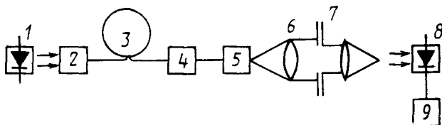
1—источник излучения; 2—устройство ввода; 3—измеряемый кабель; 4—фильтр мод оболочки; 5—устройство крепления; 6—конденсор; 7—регулируемая диафрагма; 8—приемник излучения; 9—регистрирующее устройство
