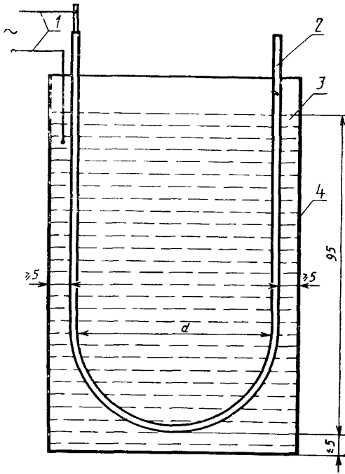
1—электроды, 2—испытуемый образец провода, 3—дробь, 4—ванна
