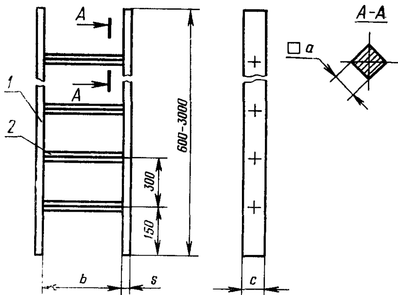
1—тетива; 2—ступенька Черт. 4
