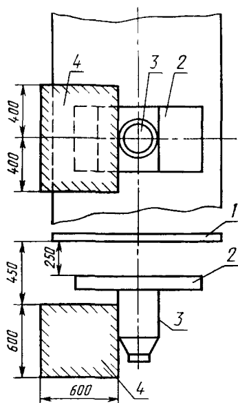
1—опорная стенка поворотного стола-штатива; 2—экрано-снимочное устройство или экранодержатель, либо панель крепления УРИ; 3—усилитель рентгеновского изображения (УРИ); 4—зона защиты.
